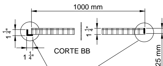
DETALHE CANTONEIRA DE AMARRAÇÃO
